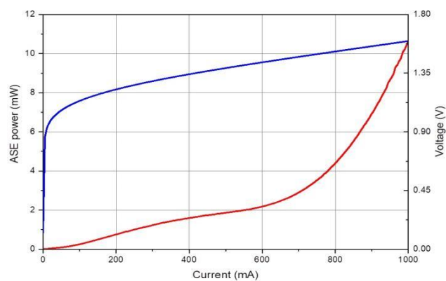
L-I-V 曲线
