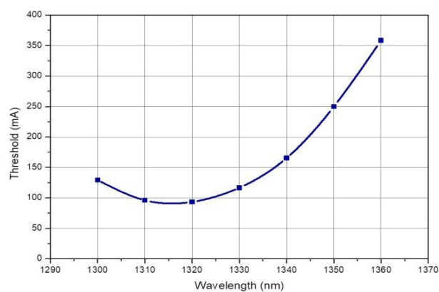
阈值电流
