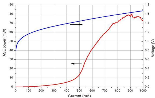
L-I-V 曲线
