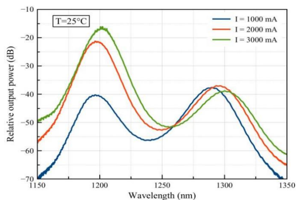
光谱(ASE)
