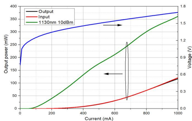
不同输入信号下的输出功率
