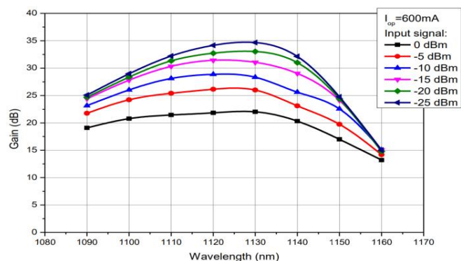
不同输入信号下的增益光谱
