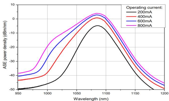
ASE 光谱 (无输入信号)
