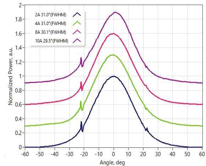
快轴远场
