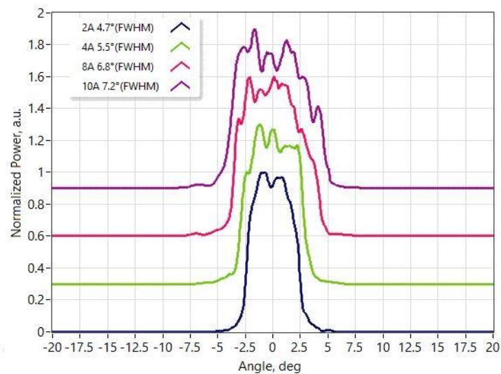
慢轴远场
