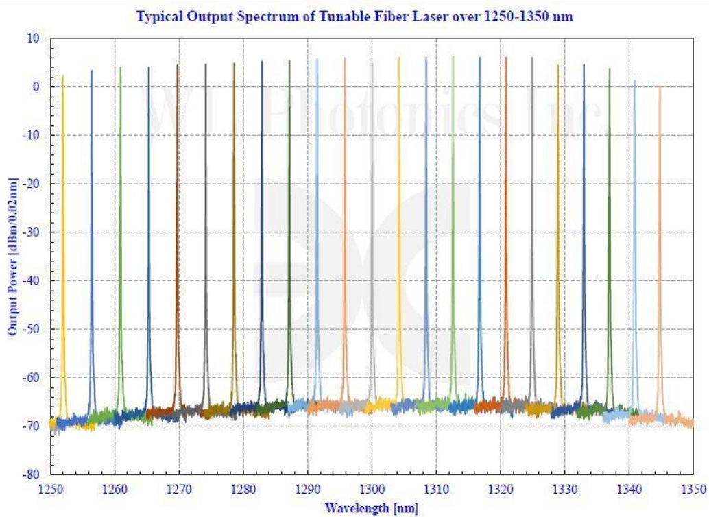
O 波段可调谐激光器的输出功率图
