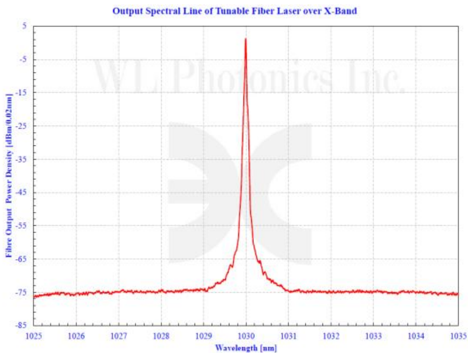
X 波段可调谐激光器输出功率图
