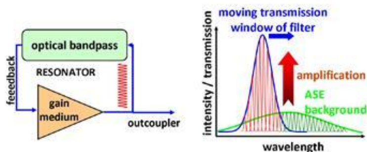
可调谐激光器的原理
