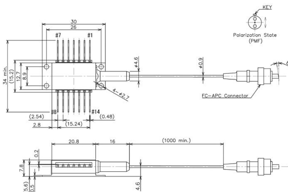
(a) 900um 光纤直径和 FC / APC 连接器类型 (QLD106L-6430)
