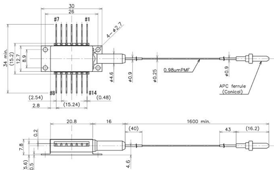
(b) 250μm 光纤直径和套圈型 (QLD106L-6430-11)
