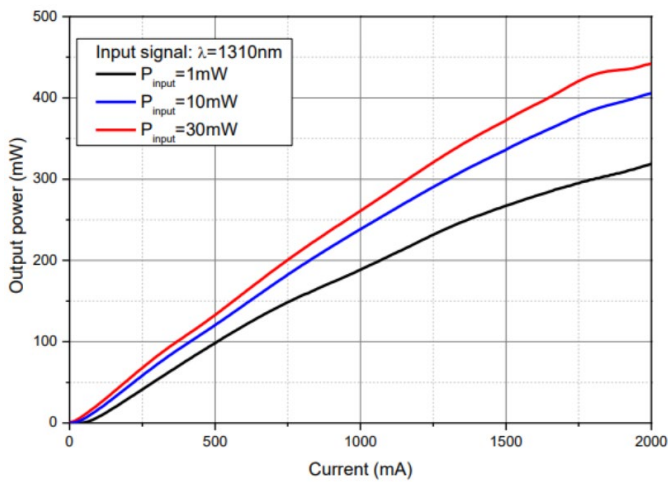
不同输入信号下的输出功率
