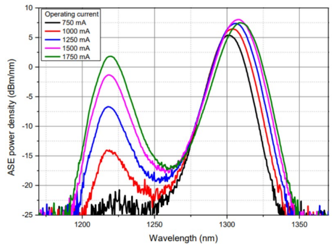
ASE光谱
