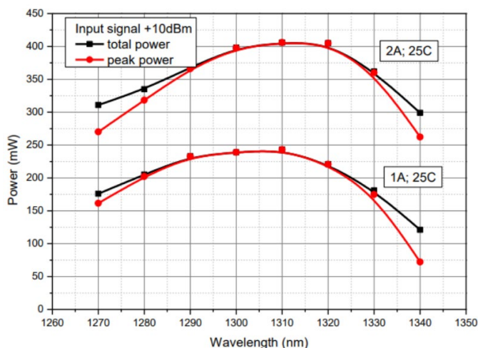
不同电流下的功率谱
