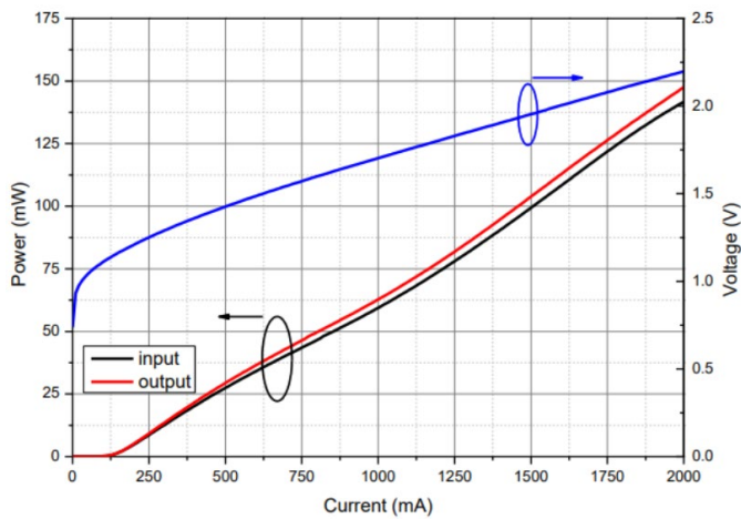
ASE LIV特性
