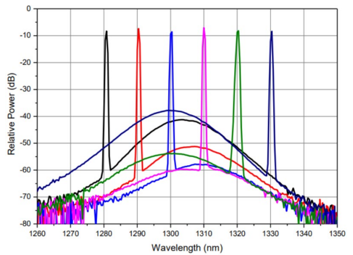
放大光信号的光谱
