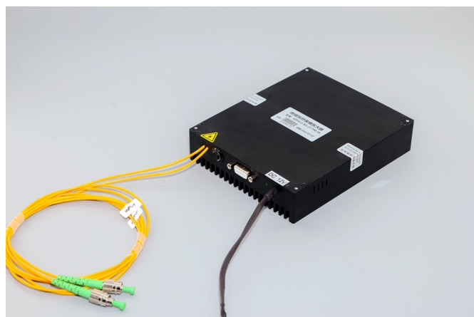
0.5W~3W高功率模块(150×125×31.5mm)
