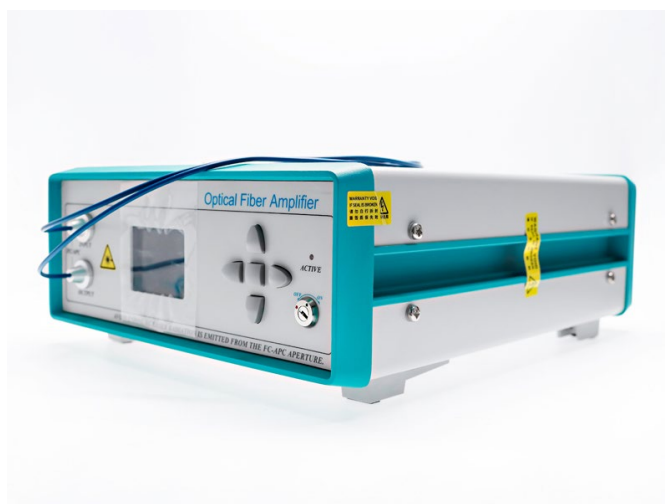
台式封装: 260(W)×320(D)×120(H)
