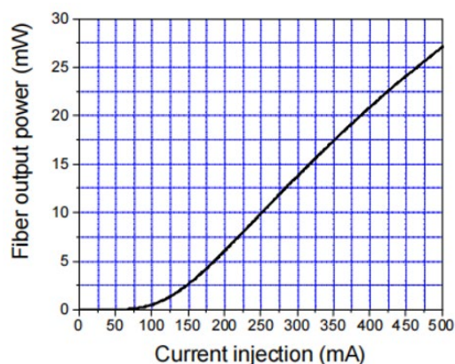
P-I 曲线
