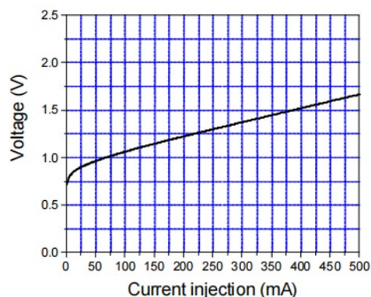
I-V 曲线
