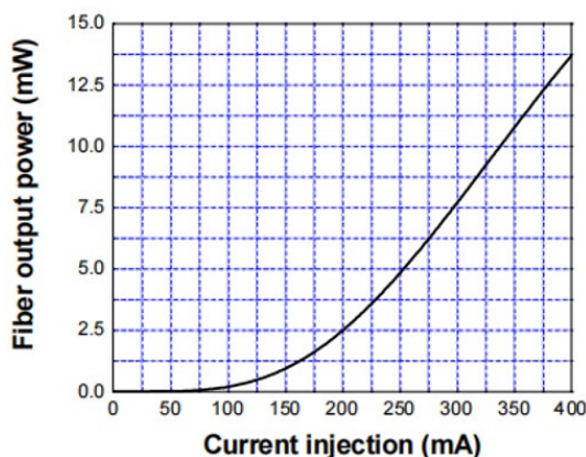
P-I 曲线
