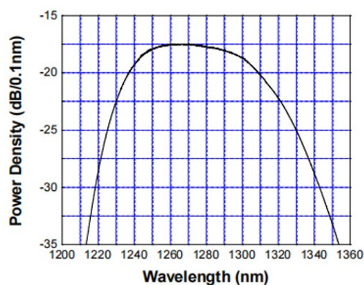
光谱图
