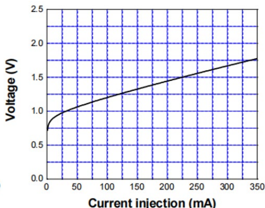
I-V 曲线
