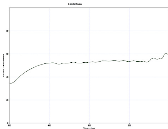
远红外透射曲线
