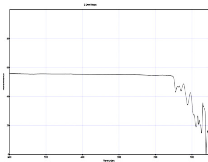
中红外透射曲线
